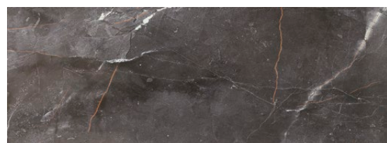
BRAINSTORM BLACK płytki ścienna | wall tile 898 x 328 x 10 mm POLYSK | GLOSS
